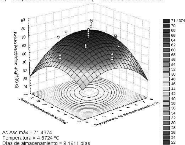
Figura 1. Superficie de respuesta para ácido ascórbico en función de temperatura de almacenamiento y tiempo en brócoli.
