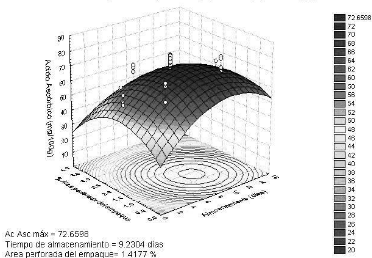
Figura 3. Superficie de respuesta para ácido ascórbico en función de tiempo de almacenamiento y porcentaje de área perforada del empaque en brócoli.
